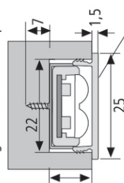
Einbau zum Schrauben mit beliebigem Standard Clip
