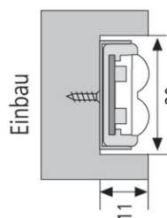
wahlweise ankleben oder anschrauben
