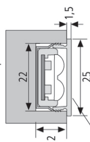
Einbau zum Klemmen mit Montageclip für Abdeckprofil
