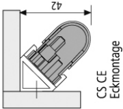
Montageanordnung mit zulässigen Abständen
