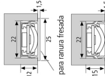
instalación para pegar con clip de montaje para perfil de cierre
